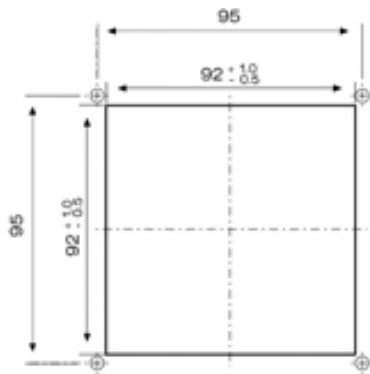
Montageausschnitt
